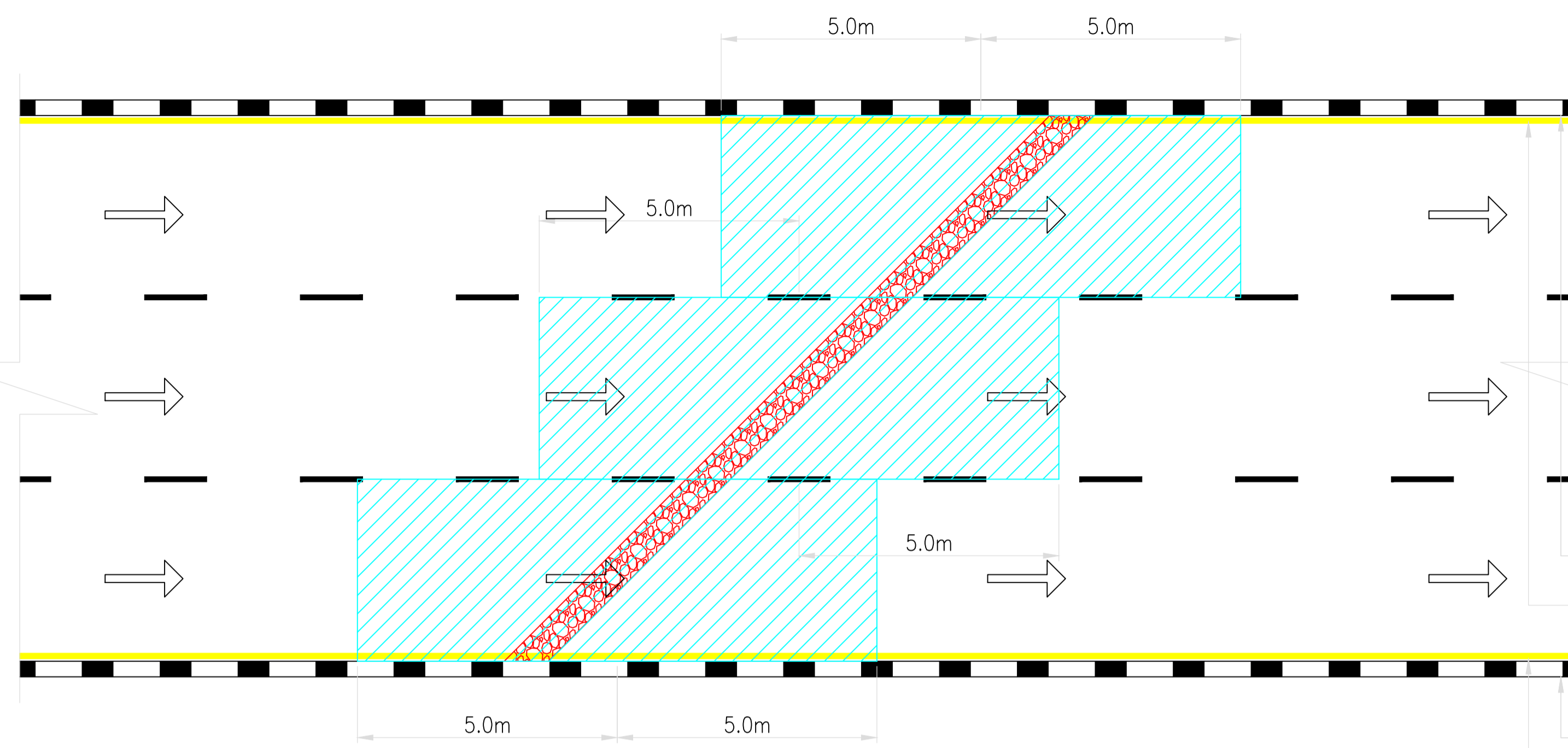
KES 8 : KOREKAN YANG MELINTANGI JALAN
