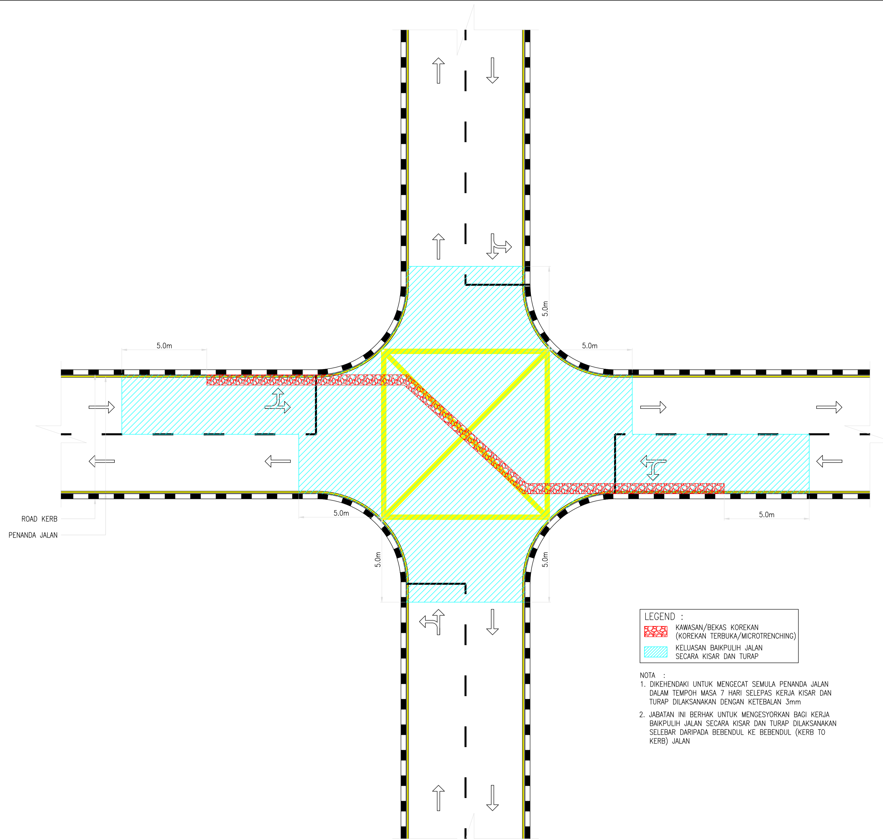
KES 10a : KOREKAN DI PERSIMPANGAN
