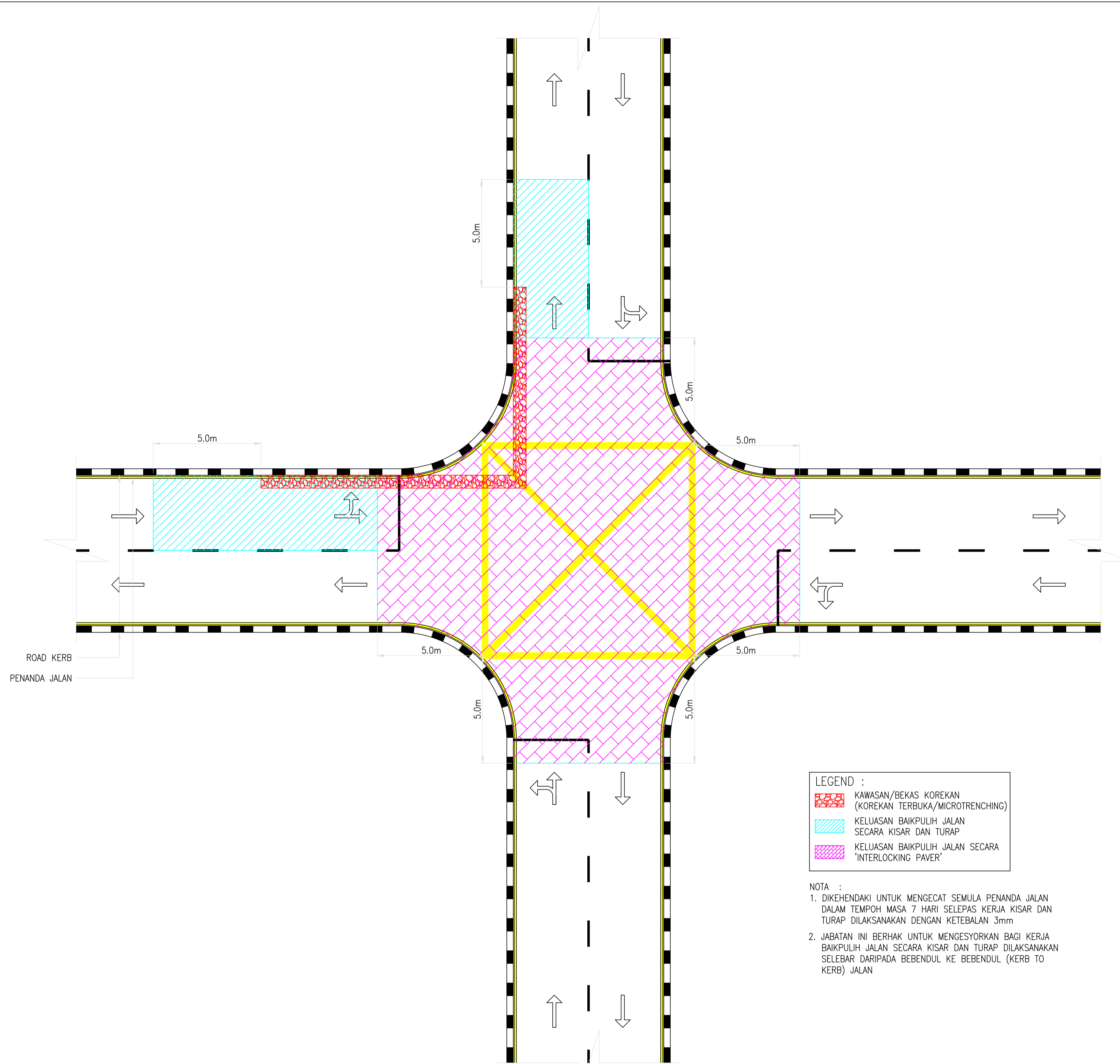
KES 1 : KOREKAN DI PERSIMPANGAN
