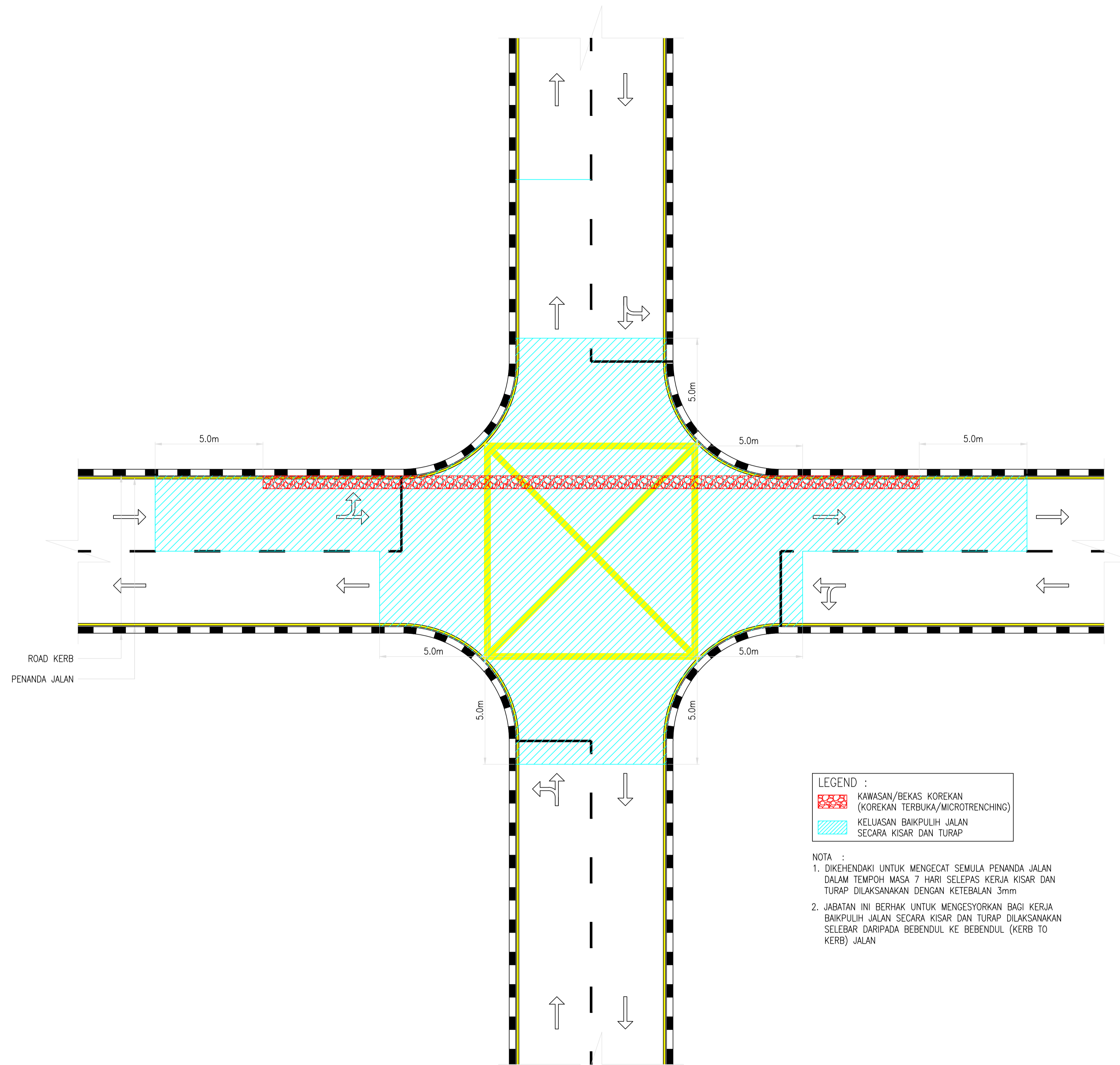
KES 10b : KOREKAN DI PERSIMPANGAN
