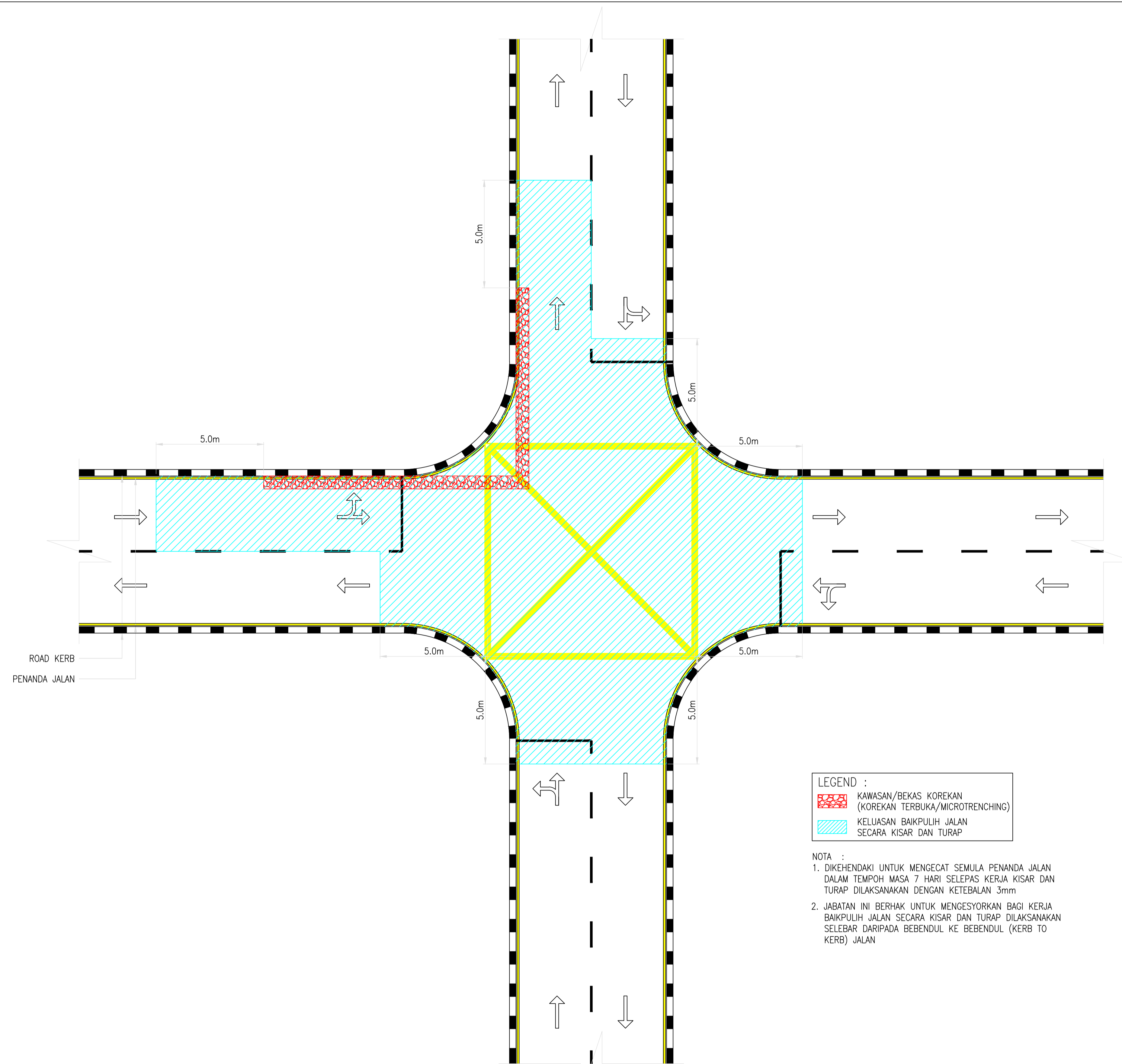
KES 10 : KOREKAN DI PERSIMPANGAN
